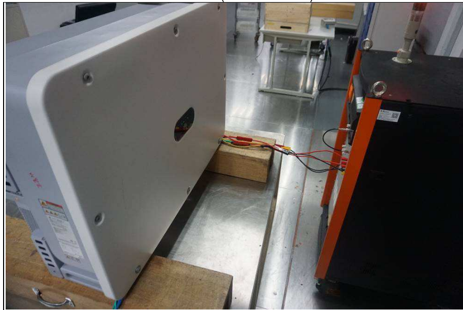
EFT TEST (AC Power Port)
